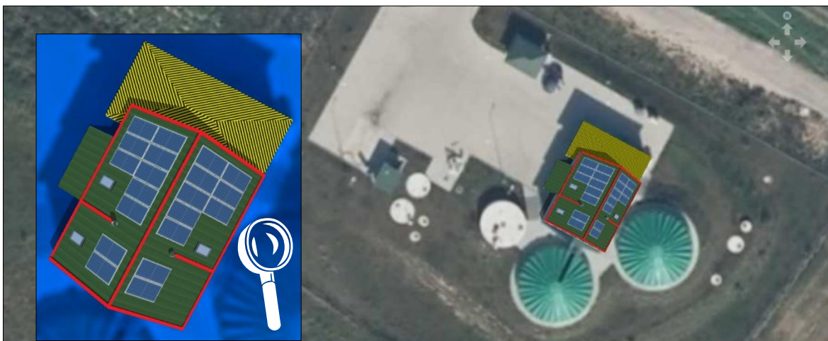
Rys. 61 Propozycja zakresu prac w ramach zamierzenia w obrębie połaci dachowych Oczyszczalni Ścieków w Sobowidzu.
