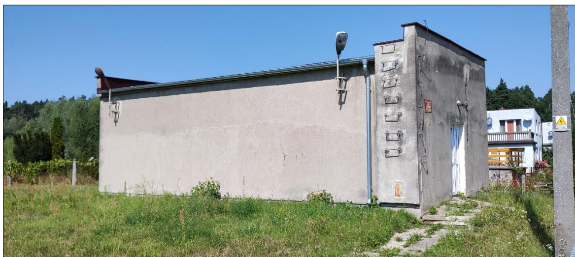
Rys. 96 Widok lokalny obiektu budowlanego Hydroforni w Sobowidzu zarejestrowany z kierunku południowego.
