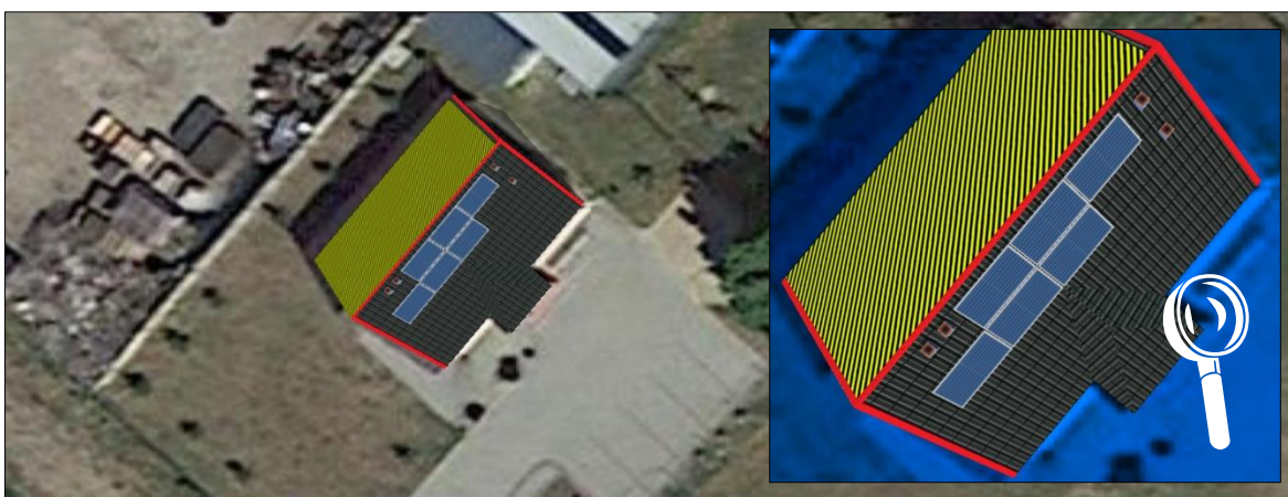
Rys. 53 Propozycja zakresu prac w ramach zamierzenia w obrębie połaci dachowych Świetlica Wiejskiej w Pawłowie.
