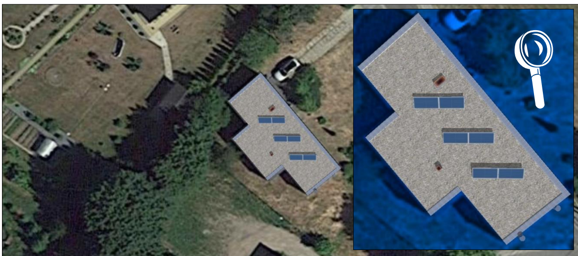
Rys. 37 Propozycja zakresu prac w ramach zamierzenia w obrębie połaci dachowych Świątlicy Wiejskiej w Kleszczewie.
